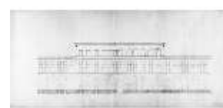
BSV-Grafikslg.IV, unausg. Entw. Hoffassade, Königsbau, ResMü., DE002335, BSV-
